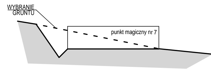
SCHEMAT FUNDAMENTY KAMIENNE GŁ. 55cm
